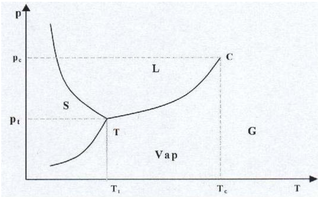
Fig. 10 Grafico p-T dell'acqua
