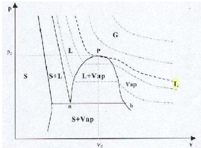
Fig. 7 Diagramma p-v dell'acqua
